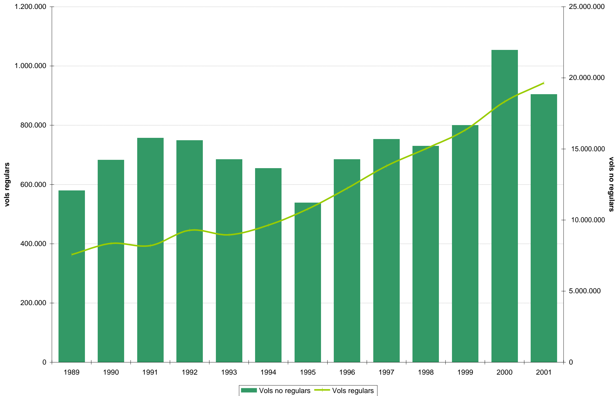
Moviment de passatgers a l'aeroport de Barcelona, 1989-2001
