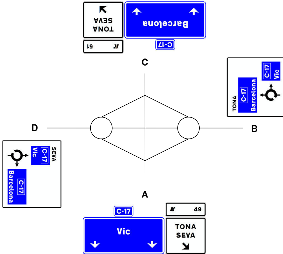
Figura 22. Senyalització resultant de l'estudi de recorreguts a la cruïlla C-17 / BV-5303
